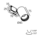
418 262 832 MDL SUPERLOOP-MIDISPY 83020 MDL
