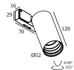
20583 9020 SUPERLOOP-SPY 52 SOFT 93020 MDL
