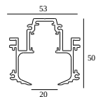
23301 0000 SPM20 - PROFILE
