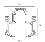
23301 0000 SPM20 - PROFILE
