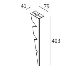
PIN 11 229 01 11
