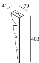
PIN 11 229 01 11
