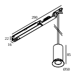
28814 9035 M - CUPPA C SOFT 93040 DIM5
