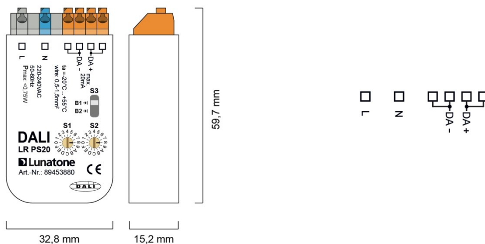
Abmessungen
