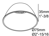
SPY 66 REFLECTOR 30° 24611 0230
