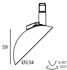
23351 9235 M20/M26H - TWEETER 92750 DIM5
