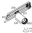
19881 9045 SPY 52 TW 96530 ADM DIM5
